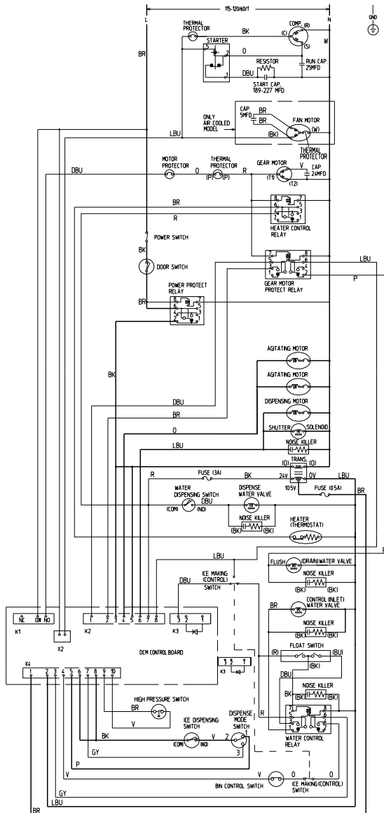
DCM-750BAH, DCM-750BWH
